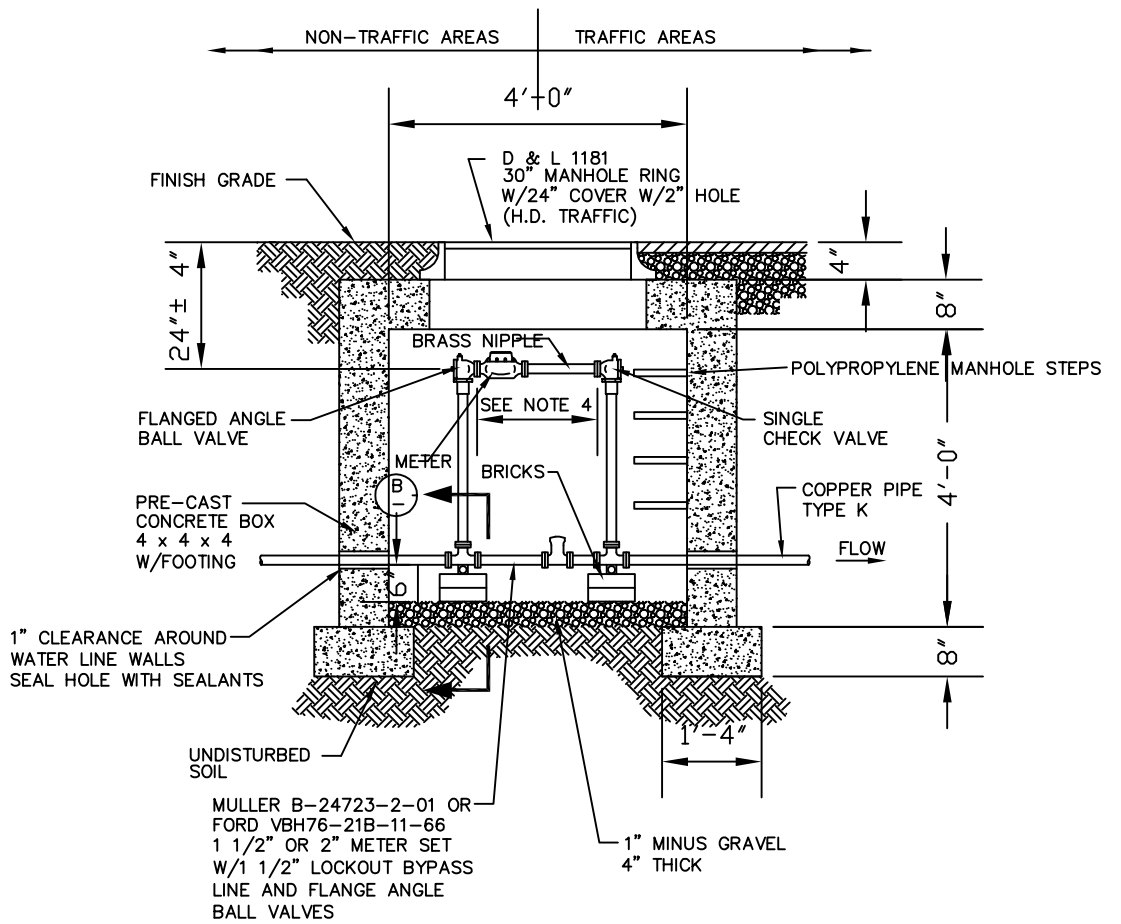
A 1 1/2" & 2" METER VAULT - N.T.S.
