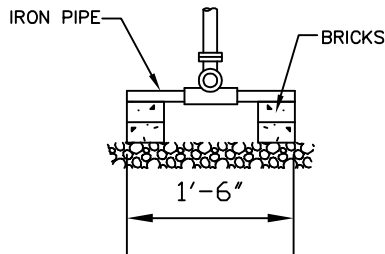
B SECTION - N.T.S.
